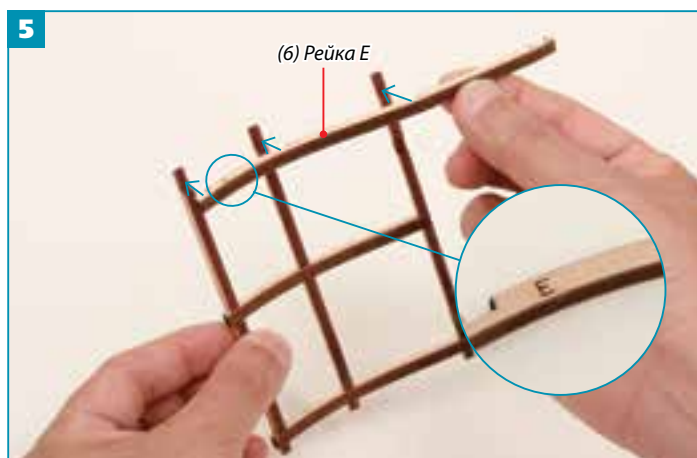
5 В верхней части вертикальных реек прикрепите при помощи клея рейку E.
