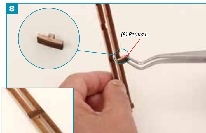
8 К средней части реек прикрепите при помощи клея рейку L.
