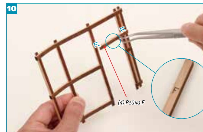
10 Переверните каркас из шага 9 и, руководствуясь фотографией, прикрепите к нему при помощи клея рейку F (места крепления см. по стрелкам).
